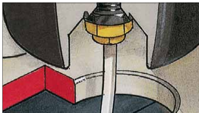
Récupération du condensat contenu dans le préfiltre.
