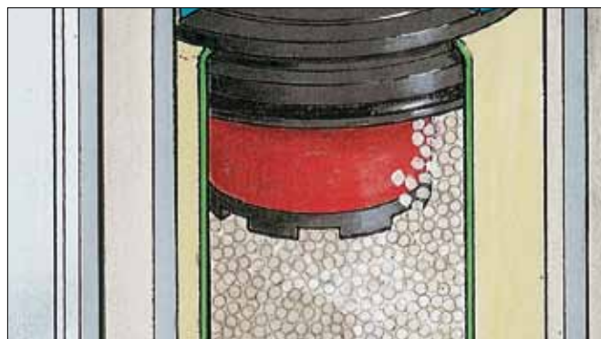
Une cartouche combinée dans chaque colonne, contenant du dessiccant DRYFIL® MS et un filtre à particules 1 µm.
