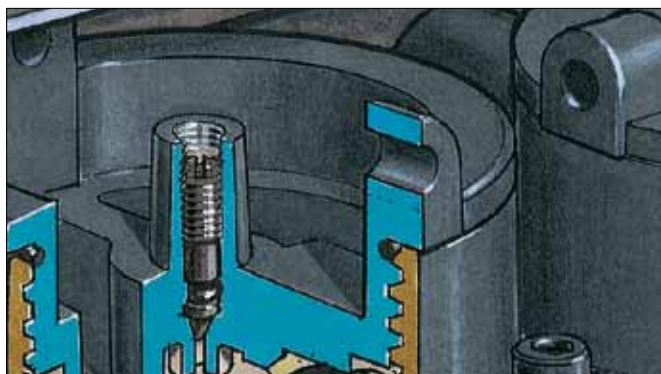
Remise en pression par le sommet pour avoir de l'air comprimé en permanence.
