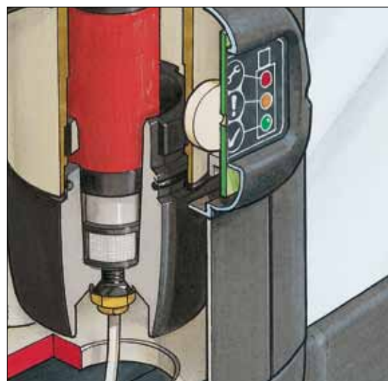
Filtre haut rendement 0,01 µm intégré.
